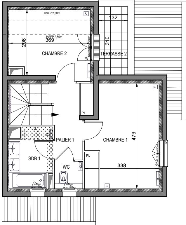
1er ETAGE
